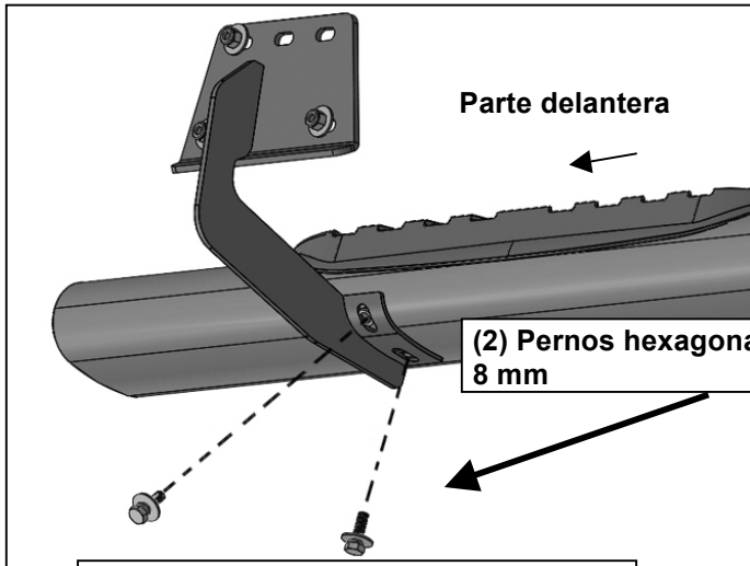
(Fig. 7) Soporte del lado delantero del pasajero fijado al estribo tubular
