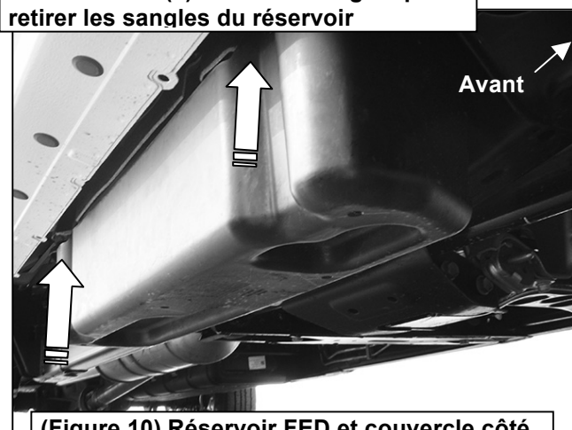
(Figure 10) Réservoir FED et couvercle côté passager
