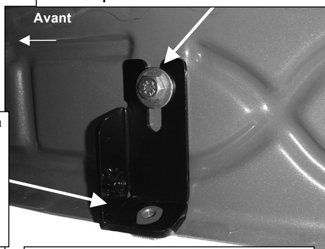
(Figure 12) Faire glisser le support supérieur sur l'écrou soudé (s'il en est équipé – voir la figure 2)
