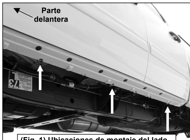
(Fig. 1) Ubicaciones de montaje del lado del conductor (3)
