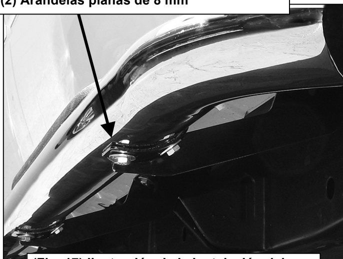
(Fig. 17) Ilustración de la instalación del lado del pasajero
