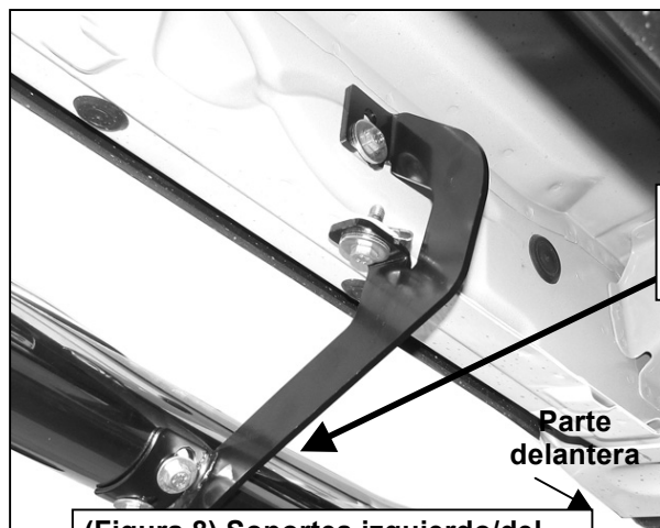
(Figura 8) Soportes izquierdo/del lado del conductor instalados
