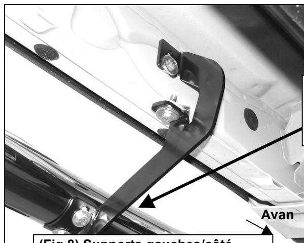
(Fig 8) Supports gauches/côté conducteur installés
