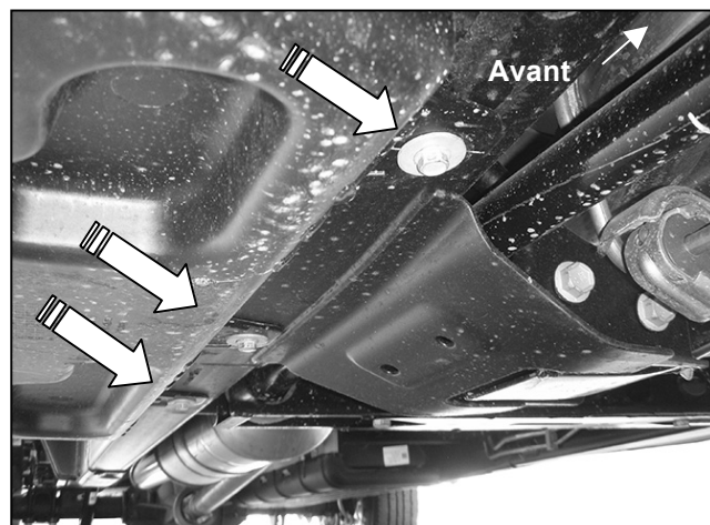
(Figure 9) Illustration de l'avant côté passager avec couvercle du réservoir FED. Démonter les (3) boulons à tête hexagonale pour retirer le couvercle
