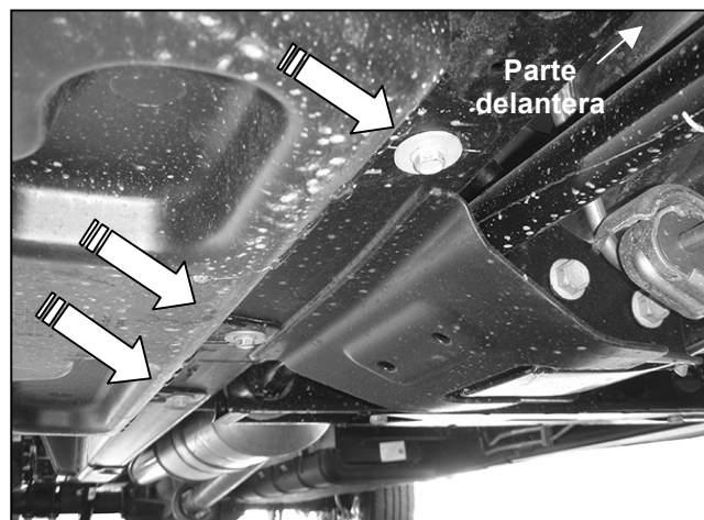
(Figura 9) Frente del lado del pasajero ilustrado con la cubierta del tanque de DEF. Retire los (3) tornillos hexagonales para extraer la cubierta
